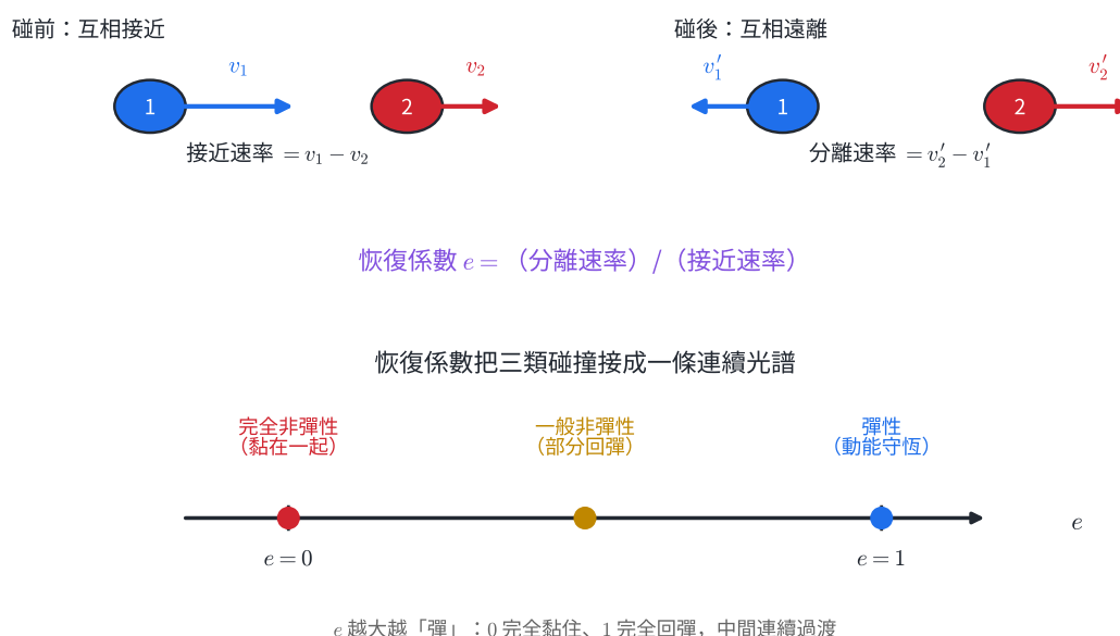
圖 1-3：恢復係數。上—— 接近速率 是碰前兩物互相靠近的相對速率 v_1 - v_2 ， 分離速率 是碰後兩物互相遠離的相對速率 v'_2 - v'_1 ，恢復係數即兩者之比。下—— e 從 0 到 1 的連續光譜： e = 0 完全非彈性（黏住）、 0 < e < 1 一般非彈性（部分回彈）、 e = 1 彈性（完全回彈、動能守恆）。
