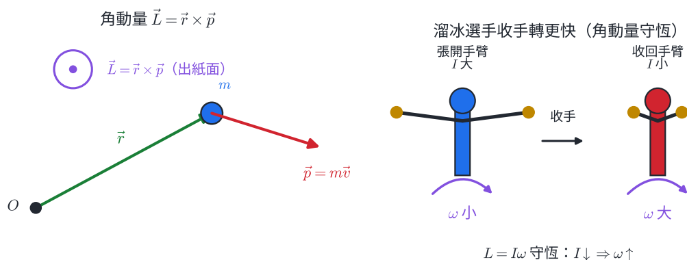
圖 1-6：左——角動量 \vec{L} = \vec{r} \times \vec{p} ，大小為 rp \sin \theta ，方向由右手定則決定（此例出紙面）。右——溜冰選手收手：質量靠近轉軸使轉動慣量 I 變小，由 L = I\omega 守恒，角速度 \omega 隨之變大。
