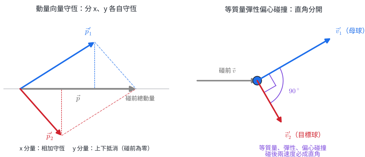
圖 1-4：二維碰撞。左——動量 向量守恆 ：碰前總動量 \vec{p} 等於碰後兩動量 \vec{p}_1' 、 \vec{p}_2' 的向量和（平行四邊形法則）；拆成分量看， x 分量相加守恆、 y 分量上下抵消（碰前 y 分量為零）。右——一動一靜、等質量的兩球作彈性偏心碰撞，碰後兩速度 \vec{v}_1' 、 \vec{v}_2' 必互相垂直（夾 90^\circ ），即撞球的直角分開現象。
